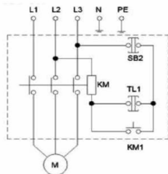
Schéma zapojenia
